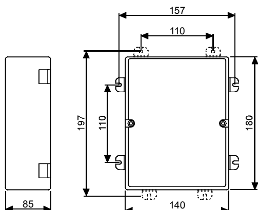
Fig.1 - DIMENSIONI (mm):
